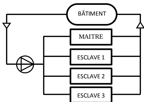
Pompe commune unique
