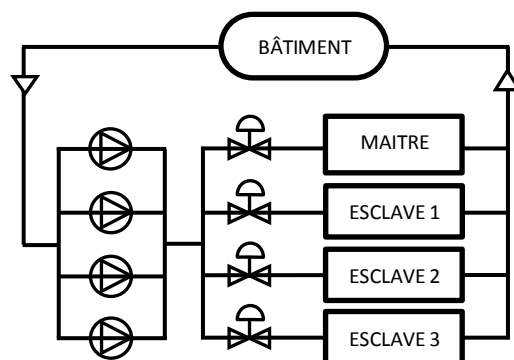
Refroidisseur avec évaporateur à sections multiples
