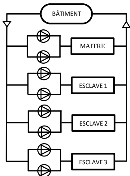
Pompe de refroidisseur double
