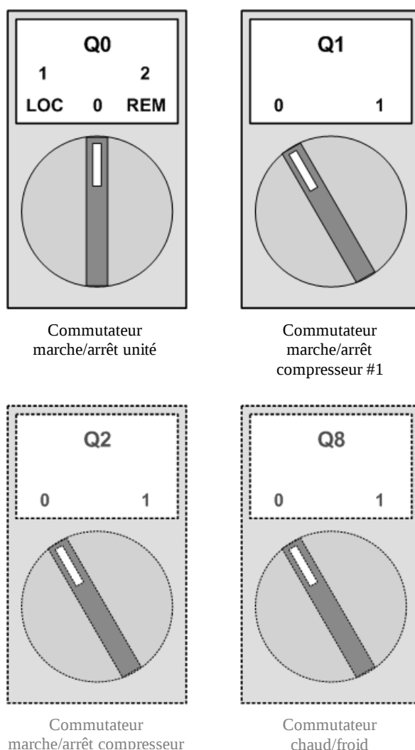
Figure 1, Commandes d'utilisation
