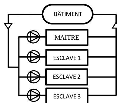
Pompe unique pour refroidisseur
