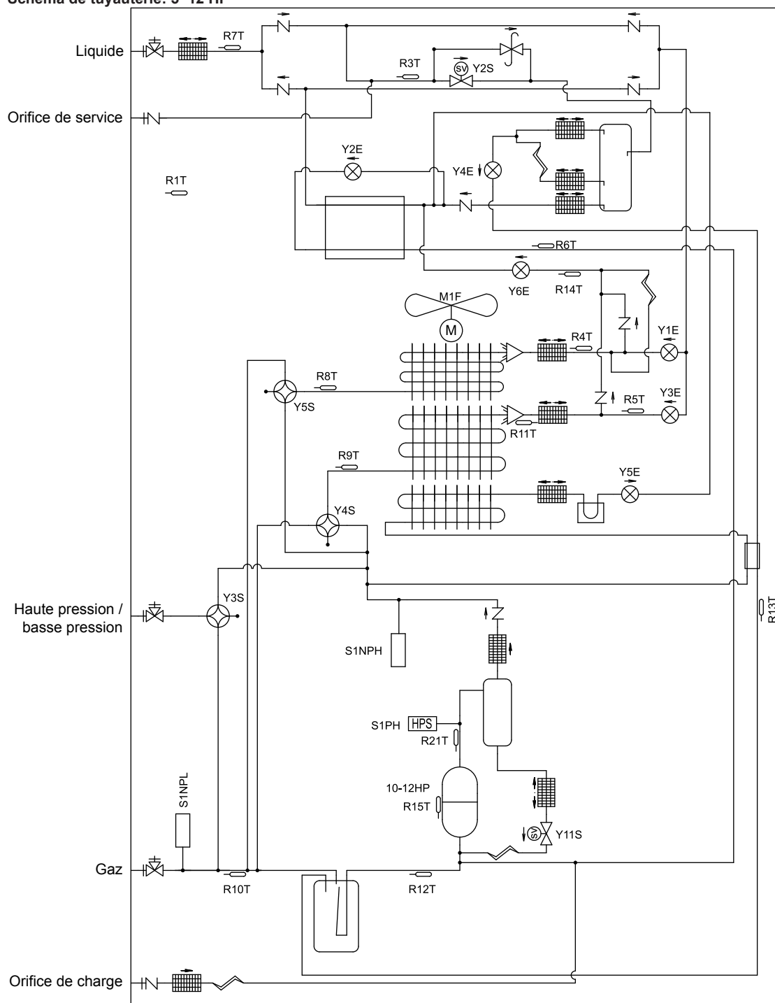
Schéma de tuyauterie: 5~12 HP
