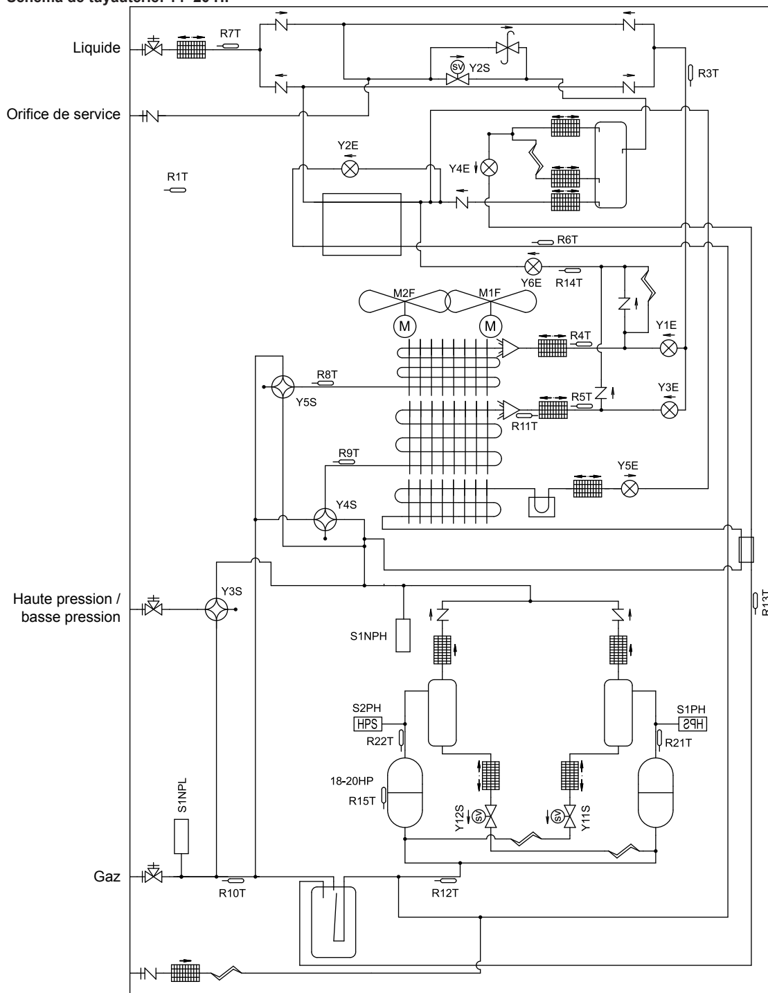
Schéma de tuyauterie: 14~20 HP
